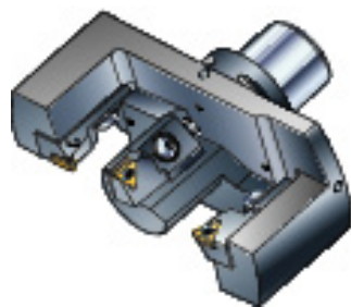
Cartuchos CoroTurn 107 de montaje axial en una herramienta de mandrinar para mecanizado interior y exterior.
