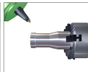
Torneado contra el husillo secundario.
