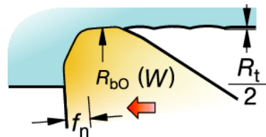
Radio Wiper igual a la velocidad de avance.
