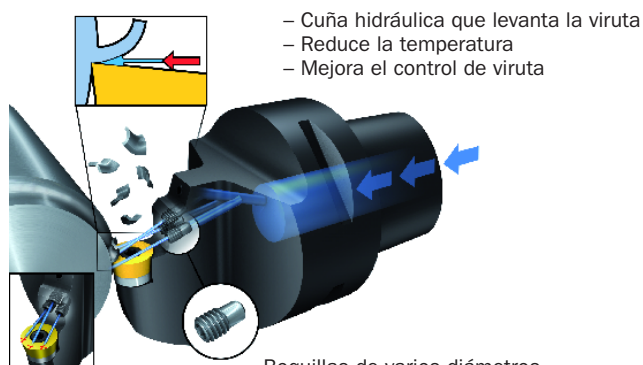
Áreas objetivo predefinidas en la cara de la plaquita
